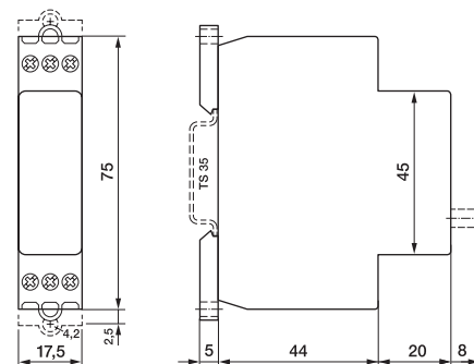
fig. 4. Dimensions (mm)
