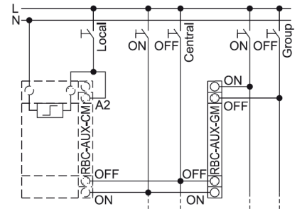
fig. 1. Wiring diagram
