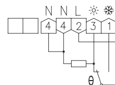
fig. 1. Wiring diagram
