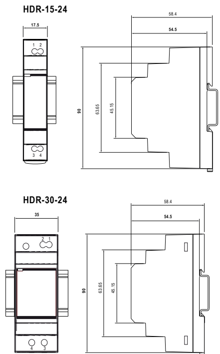
fig. 1. Dimension (mm)
