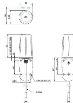
fig. 1. Dimension (mm)
