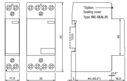
fig. 2. Abmessungen (mm)
