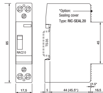
fig. 3. Abmessungen (mm)
