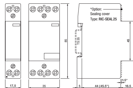
fig. 2. Abmessungen (mm)
