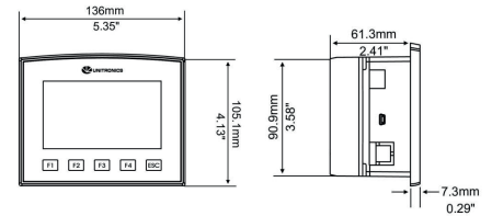
fig. 1. Dimensions (mm)
