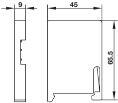
fig. 1. Dimensions (mm)
