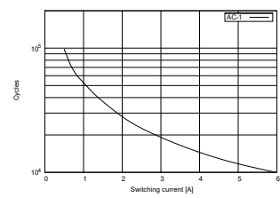
fig. 3. Gleichstrom-Grenzlastkurve
