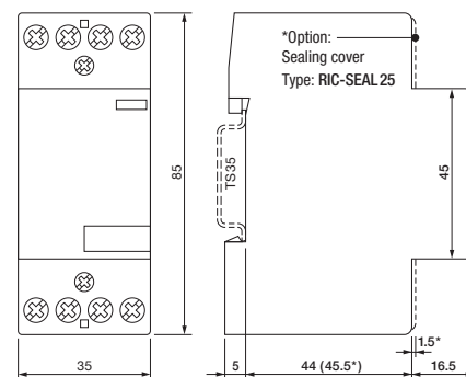
fig. 2. Abmessungen (mm)
