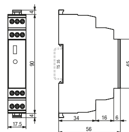
fig. 2. Abmessungen (mm)
