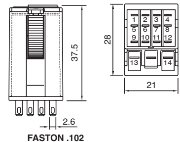
fig. 4. Abmessungen (mm)
