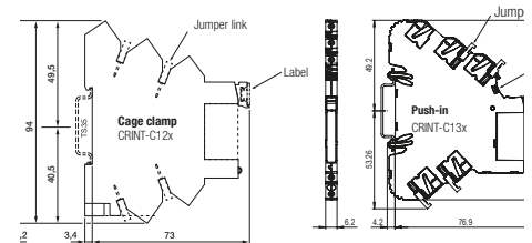
fig. 4. Dimensions (mm)
