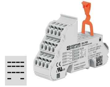
fig. 1. Wiring diagram
