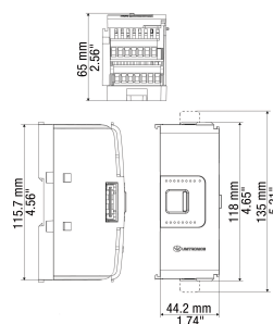
fig. 1. Abmessungen (mm)
