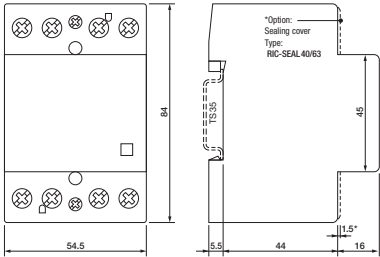
fig. 3. Dimensions (mm)
