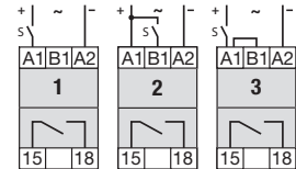
fig. 2. Wechselstrom-Schaltzyklen
