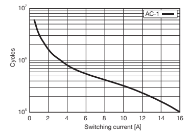
fig. 2. Wechselstrom-Schaltzyklen
