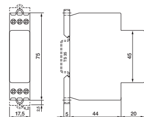
fig. 4. Abmessungen (mm)
