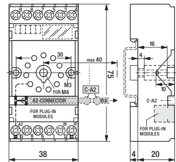
fig. 2. Abmessungen (mm)
