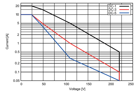
fig. 2. Gleichstrom-Grenzlastkurve
