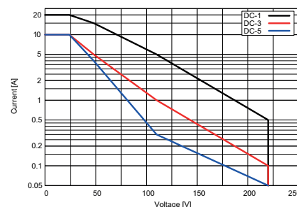
fig. 2. Gleichstrom-Grenzlastkurve
