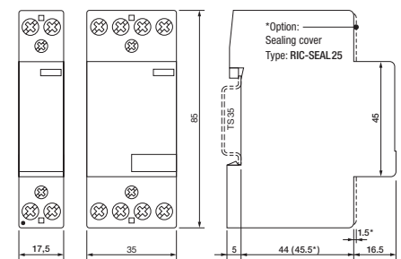
fig. 3. Abmessungen (mm)
