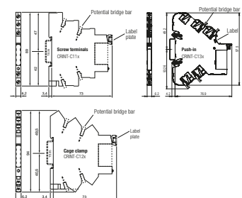
fig. 4. Abmessungen (mm)
