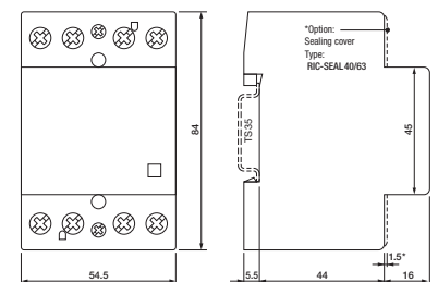
fig. 3. Abmessungen (mm)
