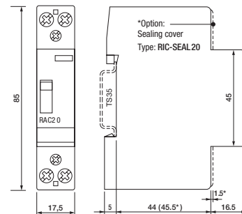
fig. 3. Abmessungen (mm)
