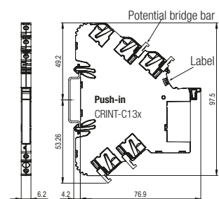
fig. 4. Dimensions (mm)
