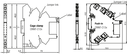
fig. 3. Dimensions (mm)
