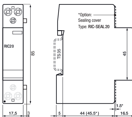
fig. 3. Dimensions (mm)
