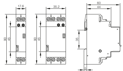
fig. 3. Abmessungen (mm)
