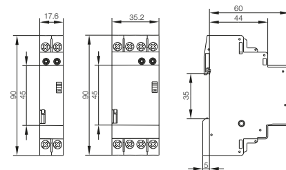
fig. 3. Abmessungen (mm)
