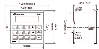
fig. 1. Abmessungen (mm)
