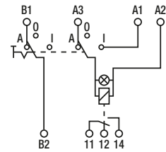
fig. 1. Verdrahtungsdiagramm
