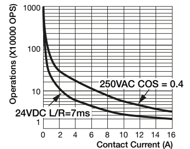
fig. 3. Gleichstrom-Grenzlastkurve
