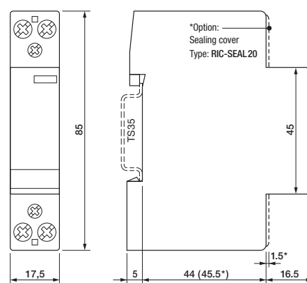
fig. 3. Dimensions (mm)
