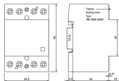
fig. 3. Abmessungen (mm)
