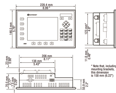
fig. 1. Dimensions (mm)
