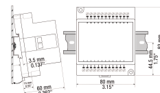
fig. 1. Abmessungen (mm)
