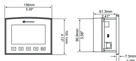
fig. 1. Dimensions (mm)
