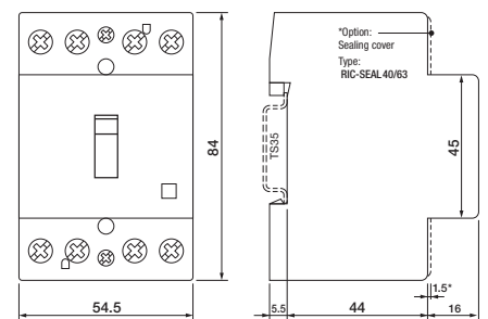
fig. 3. Abmessungen (mm)
