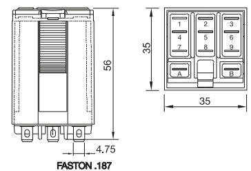
fig. 4. Dimensions (mm)
