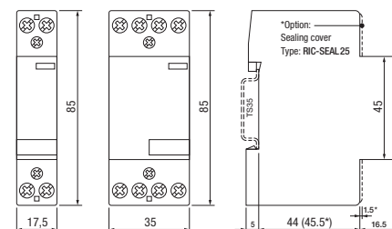
fig. 3. Abmessungen (mm)
