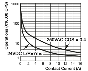
fig. 3. Gleichstrom-Grenzlastkurve
