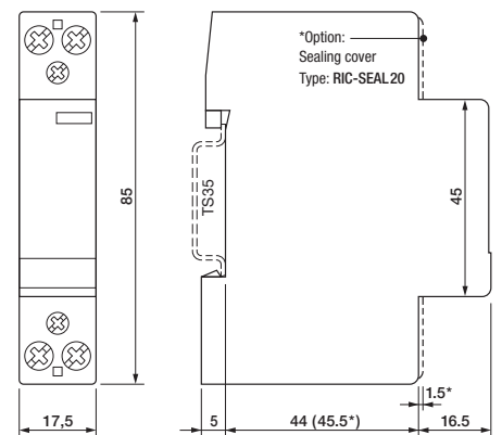
fig. 3. Abmessungen (mm)
