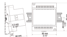
fig. 1. Abmessungen (mm)
