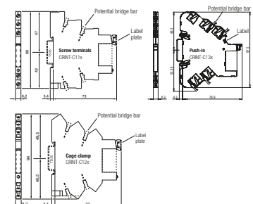
fig. 4. Abmessungen (mm)
