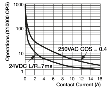
fig. 3. Gleichstrom-Grenzlastkurve
