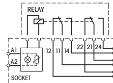
fig. 2. Wechsel-/Gleichstrom-Schaltzyklen
