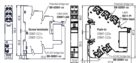
fig. 4. Abmessungen (mm)
