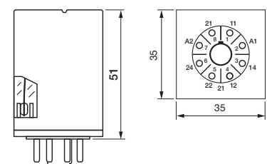
fig. 4. Dimensions (mm)
