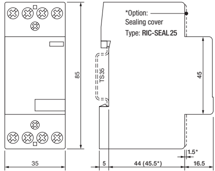
fig. 3. Dimensions (mm)
