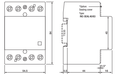
fig. 3. Dimensions (mm)
