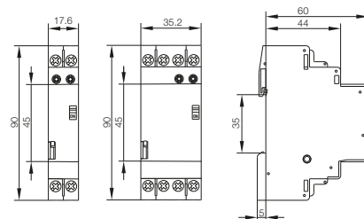
fig. 3. Dimensions (mm)
