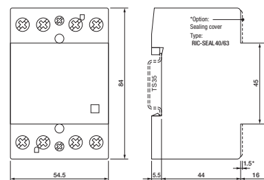
fig. 3. Dimensions (mm)
